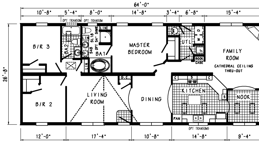
CN131-A 2864 Approx. 1707 Sq. Ft.
